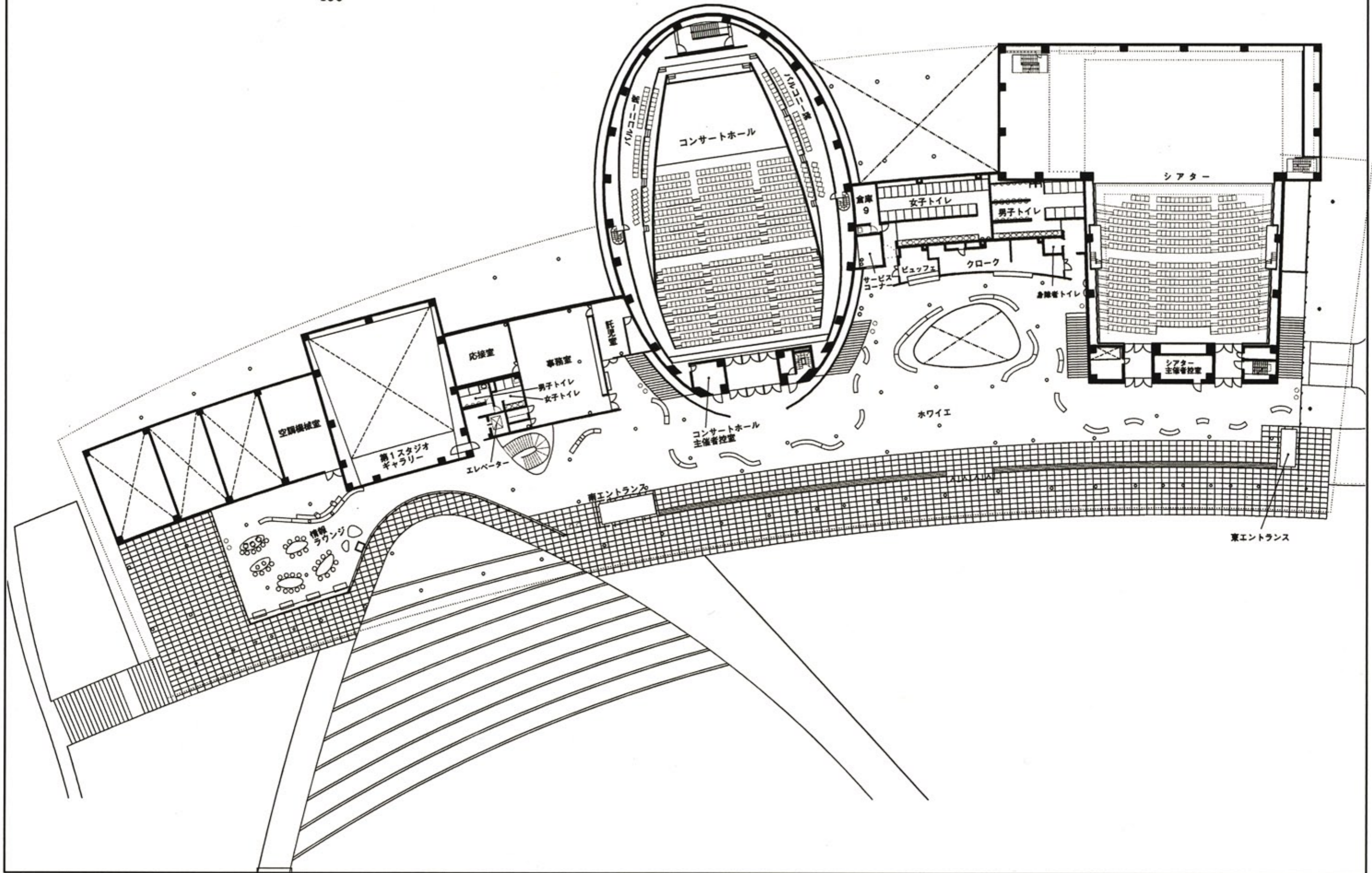
長岡リリックホール 2F平面図 \frac{1}{400}
